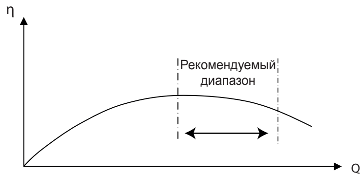
Кривая производительности насоса
