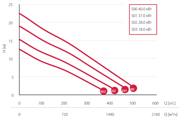
DN300
